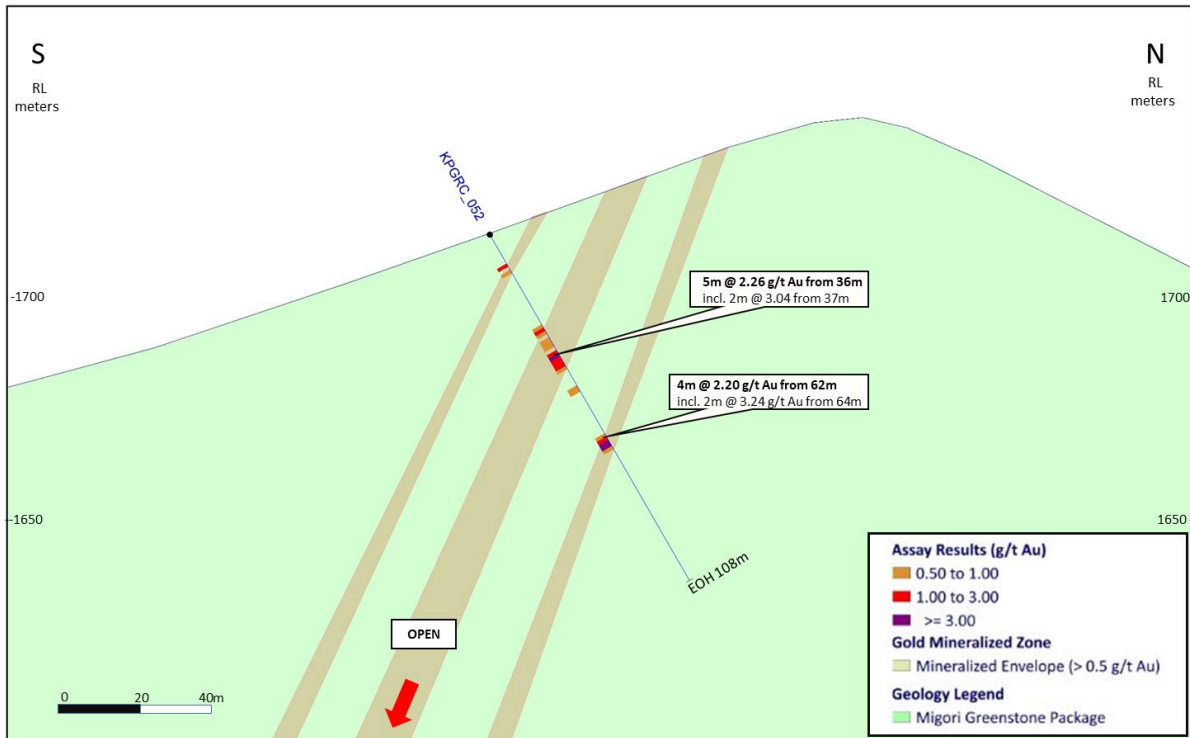
Profilschnitt Süd-Nord - Bohrung KPGRC 052
