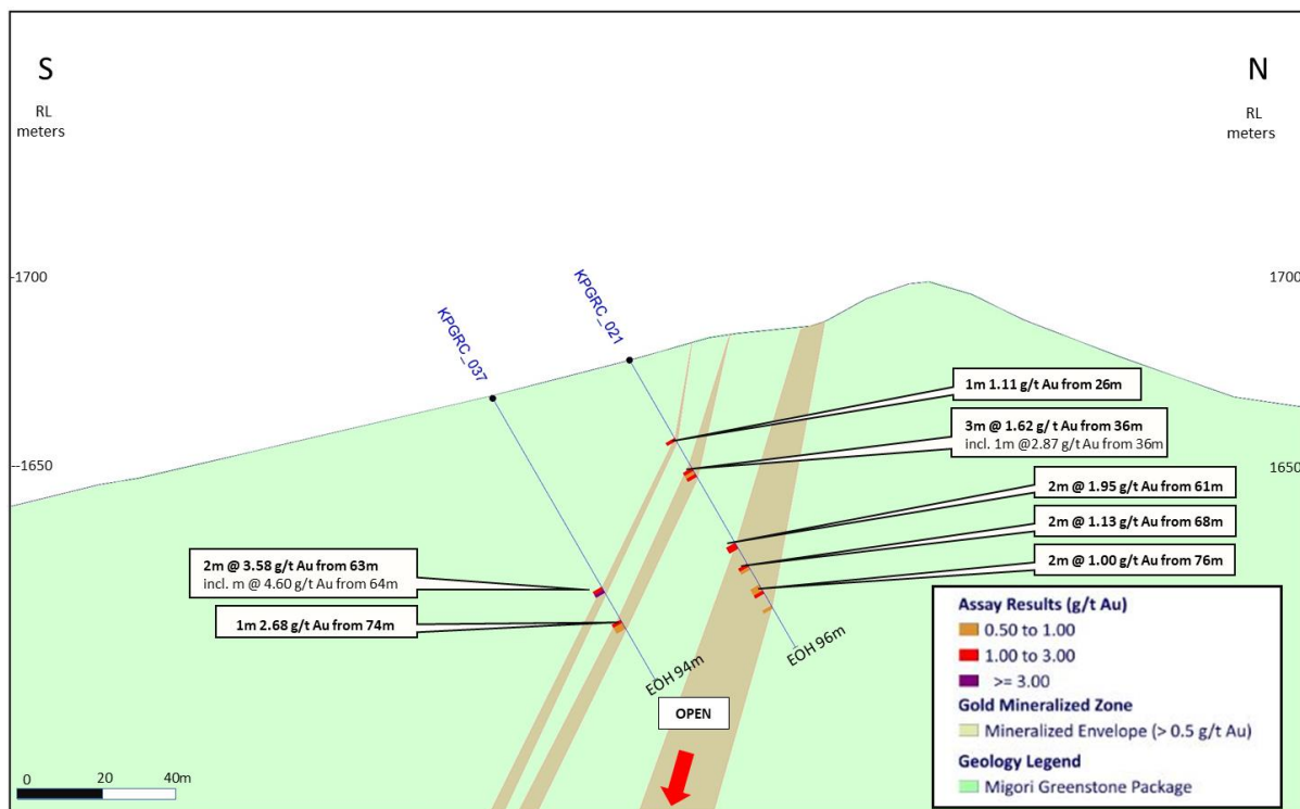
Profilschnitt Süd-Nord - Bohrungen KPGRC 021 und KPGRC 037
