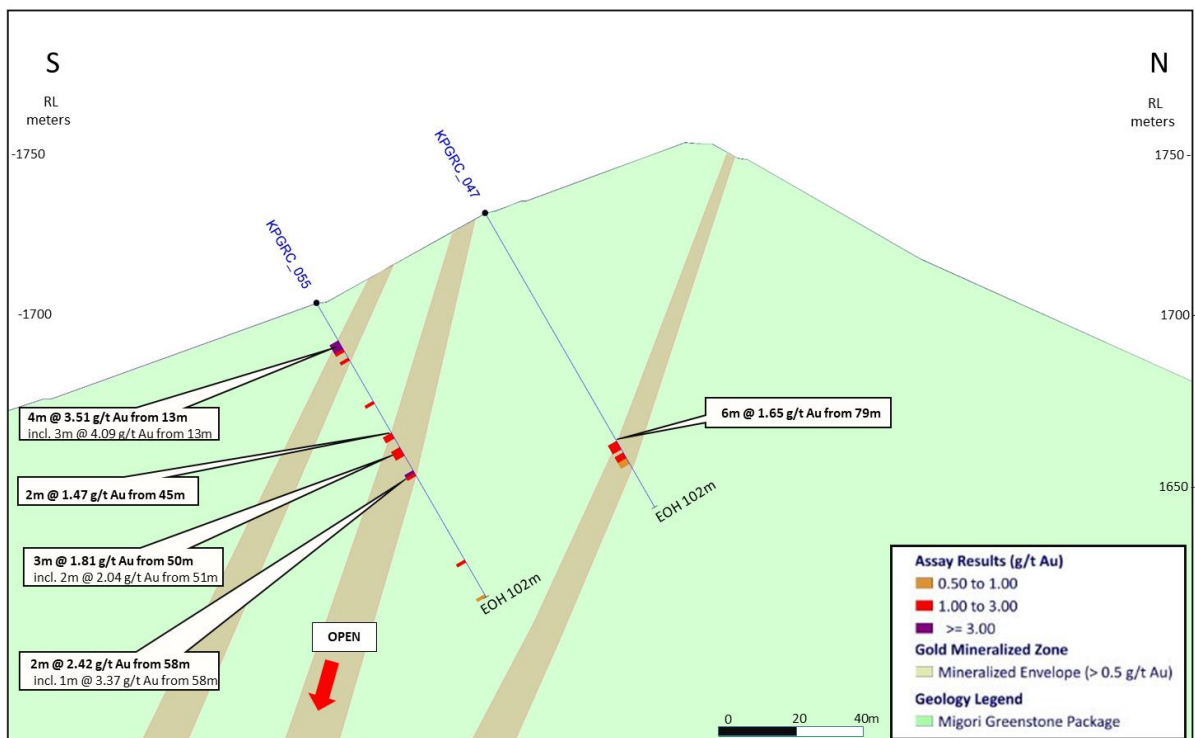
Profilschnitt Süd-Nord - Bohrungen KPGRC 055 und KPGRC 047
